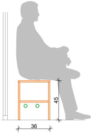
Ülőpad metszete
