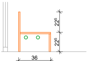
Gyerek ülőpad metszete
