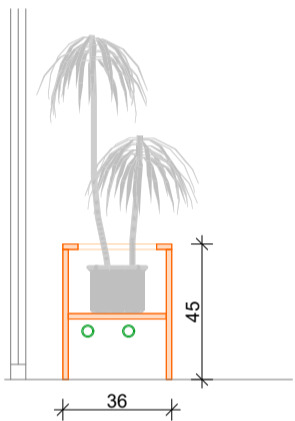
Növényláda metszete
