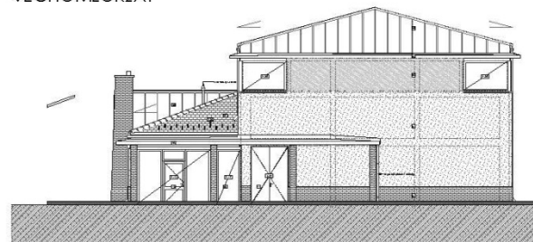
VÉGHOMLOKZAT
