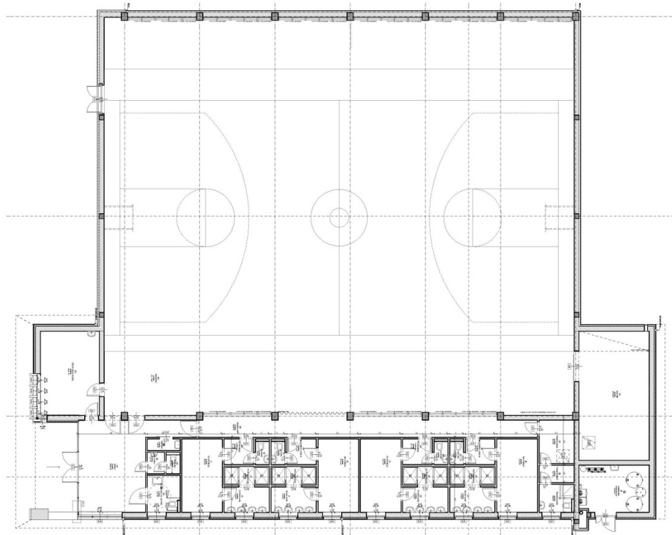
ALAPRAJZ
