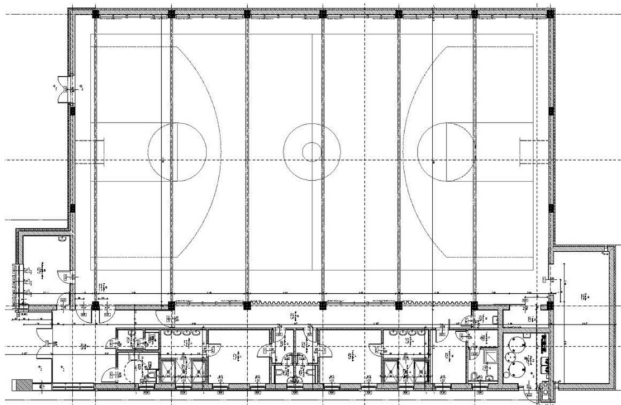
ALAPRAJZ
