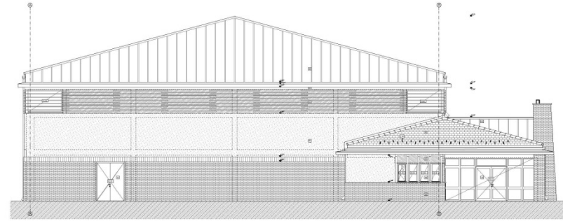
VÉGHOMLOKZAT
