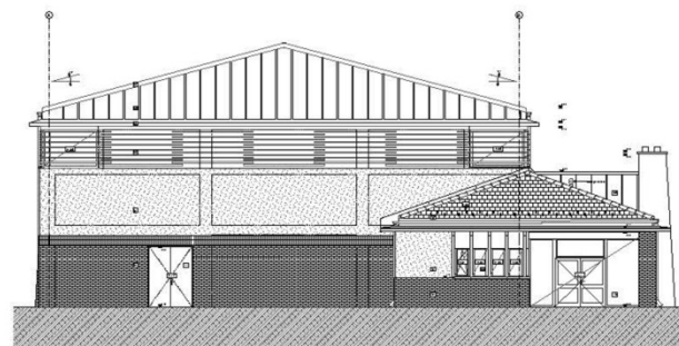
VÉGHOMLOKZAT
