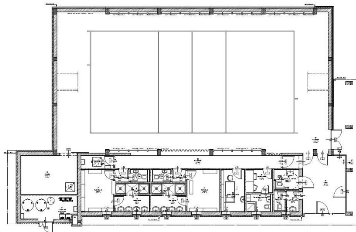
ALAPRAJZ
